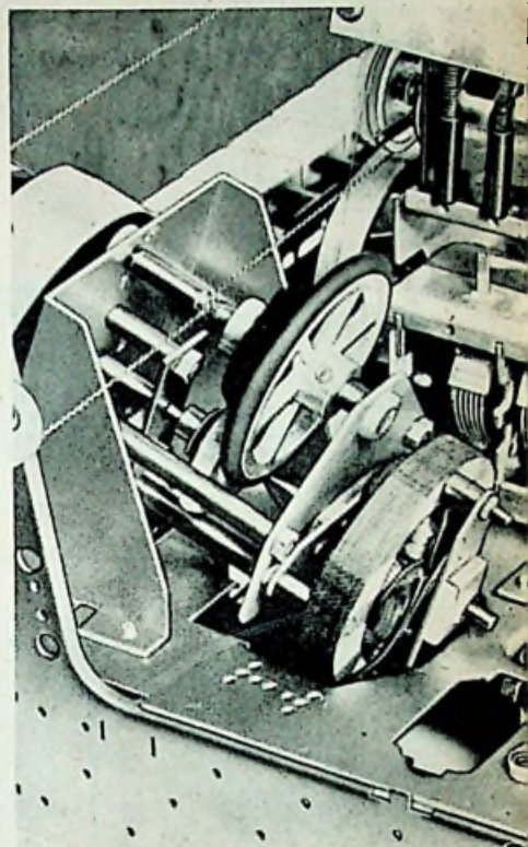
Motoraandrijfsmechanisme bij de Grundig-apparaten 4040 W/3D, 5040 W/3D en 5050 W/3D
